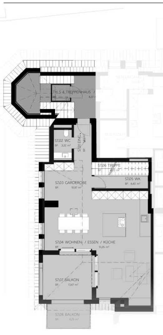
4. OG | Attika
