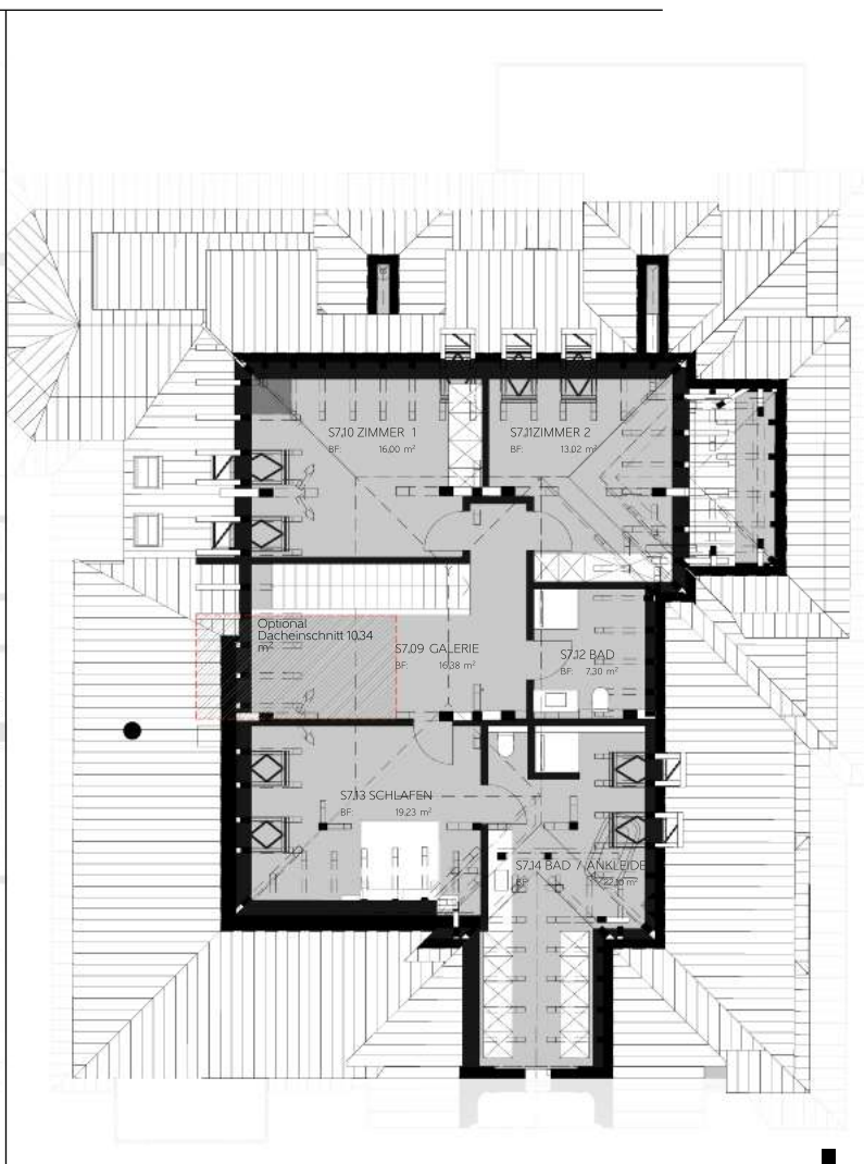
4. OG | Attika
