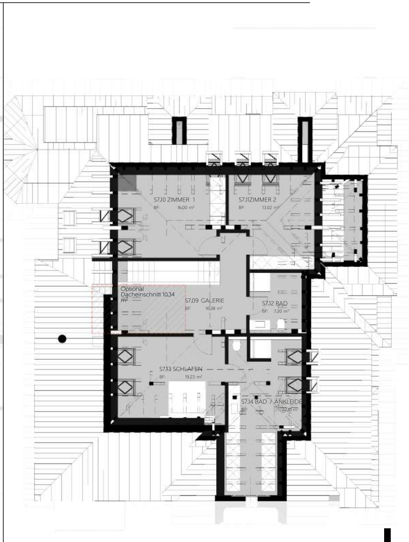
4. OG | Attika
