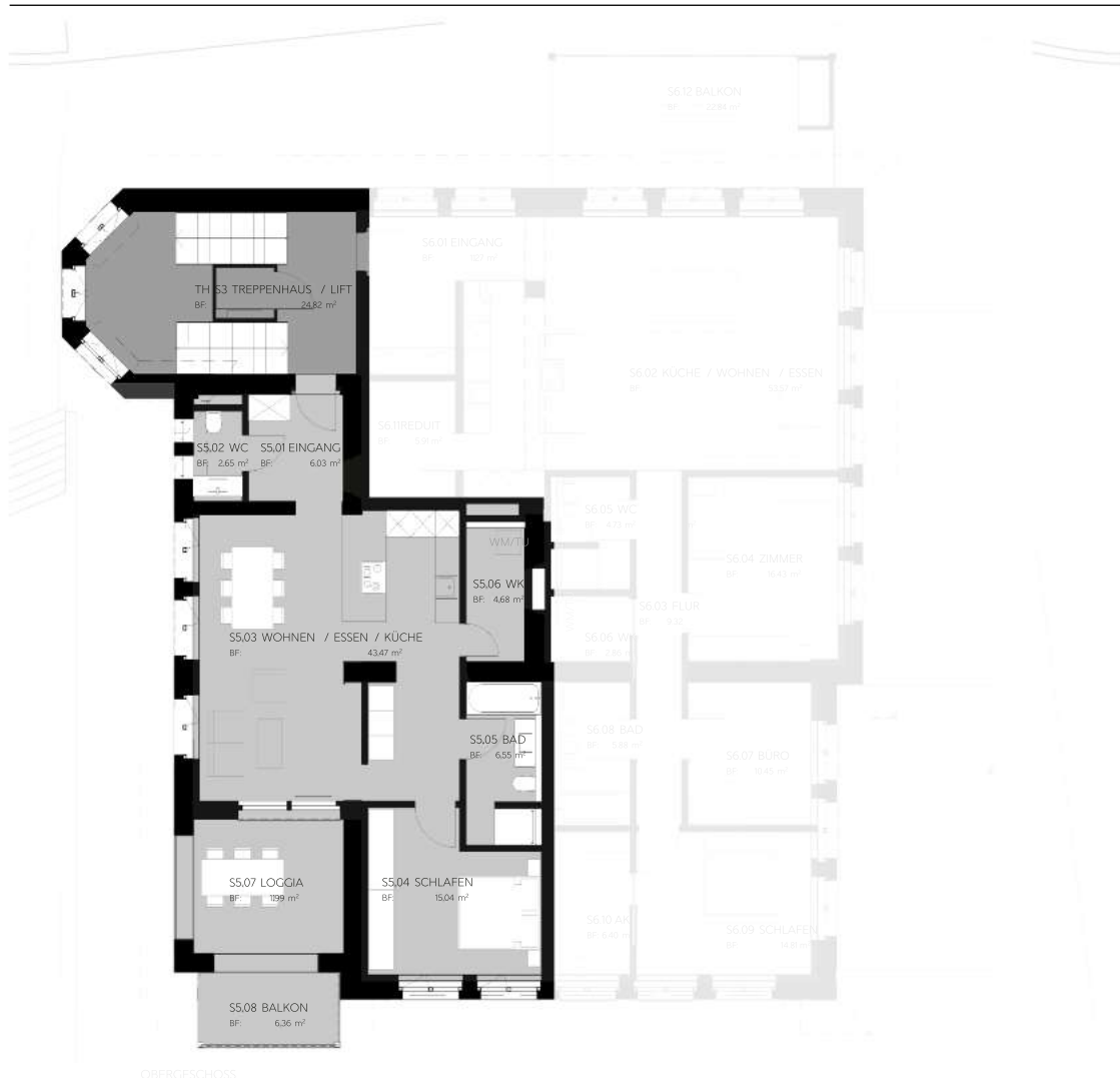
OBERGESCHOSS
